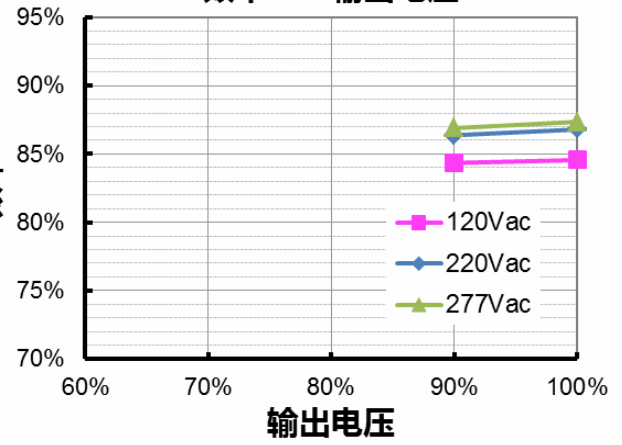
LUR-040S150ST( I_o=1500mA ) 效率 vs. 输出电压
