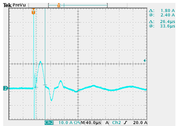
EDC-075S105ST( I_o=1050\text{mA} )
